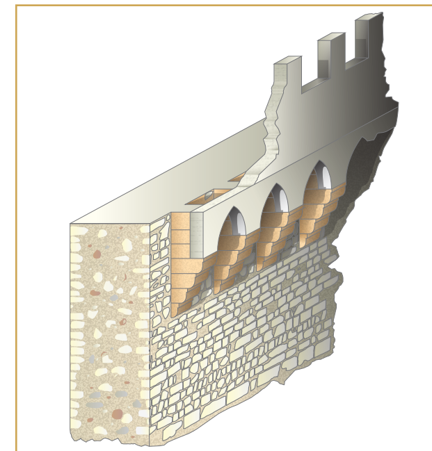
535 Restitution du crénelage de la tour Bellegarde d'après les vestiges.
